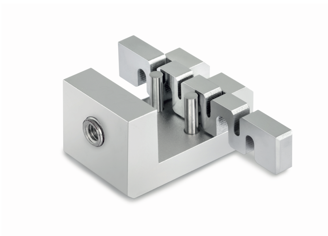
Borne d'arrachage de câble
