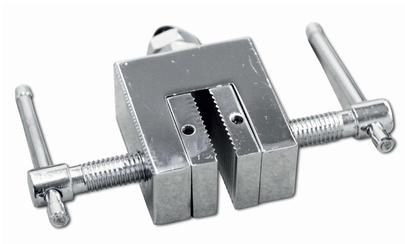
Pince universelle à mâchoire double pour tests de traction et de déchirement
